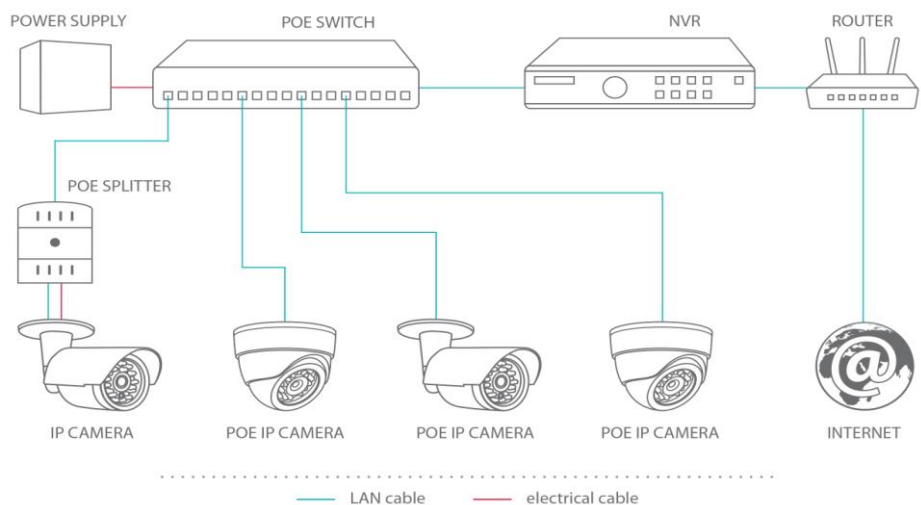
Схема підключення:
